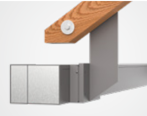
Dakspantmontage
