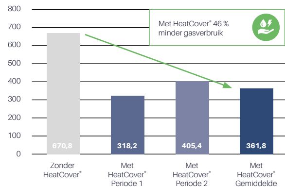
GASVERBRUIK ZONDER VS MET HEATCOVER® IN M³ PER WEEK
