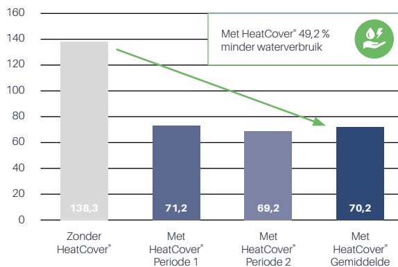
WATERVERBRUIK ZONDER VS MET HEATCOVER® IN M³ PER WEEK
