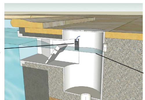
Plaatsing van de sonde in de skimmer
